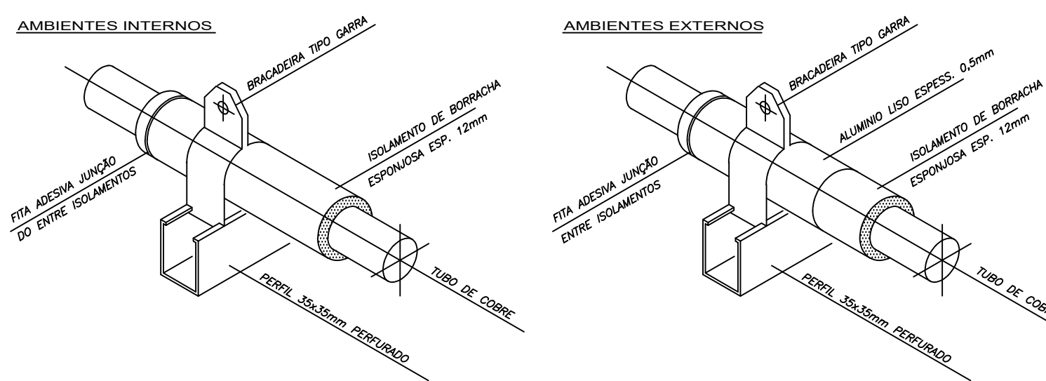
DET. SUPORTE TUBULAÇÃO FRIGORÍGENA
