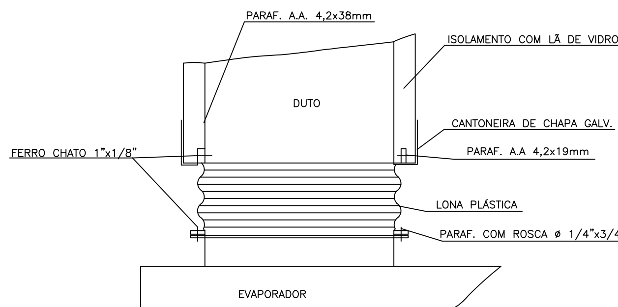
DETALHE CONEXÃO EQUIPAMENTO
