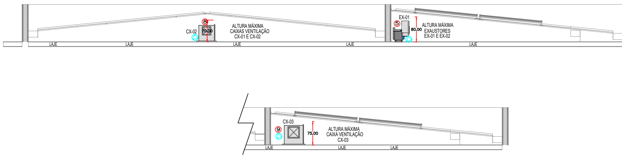
DETALHE ALTURA MÁXIMA EQUIPAMENTOS VENTILAÇÃO
