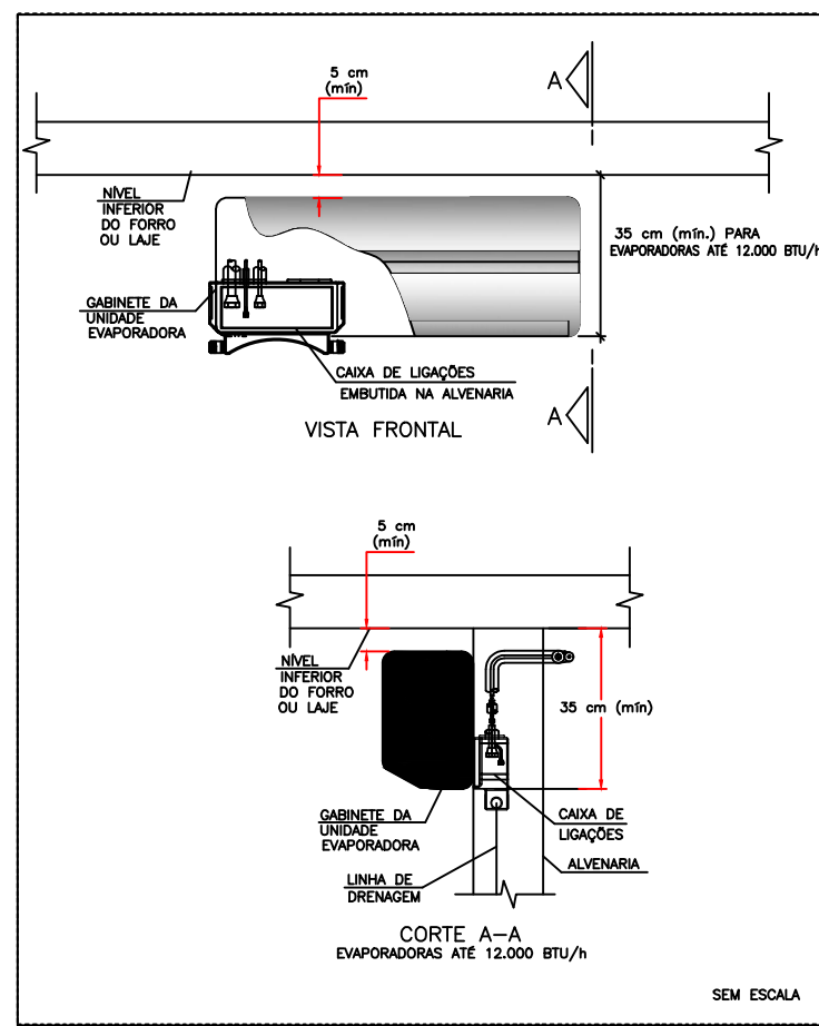
CAIXA DE LIGAÇÕES
