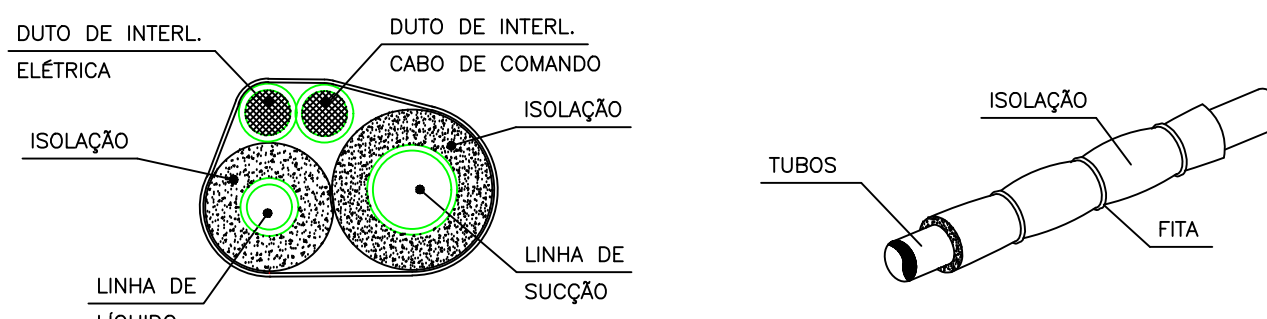
DET. ISOLAÇÃO TUBULAÇÃO FRIGORÍGENA
