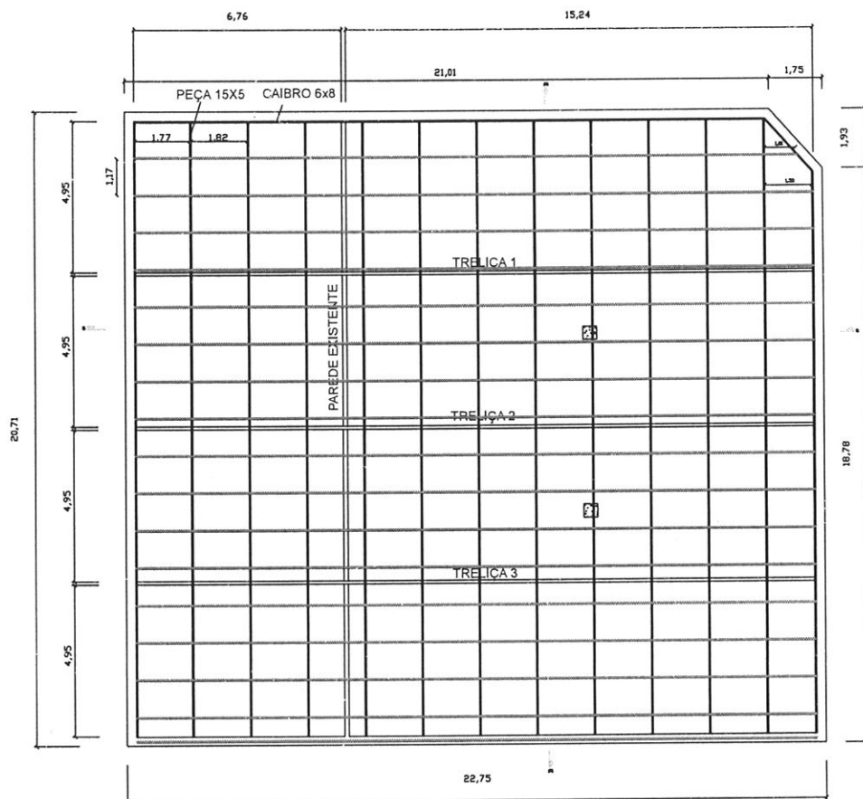
PLANTA BAIXA DA ESTRUTURA DO TELHADO
