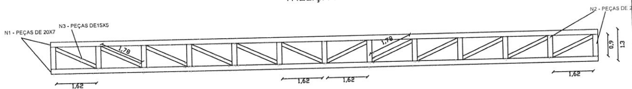
TRELÇA 1
