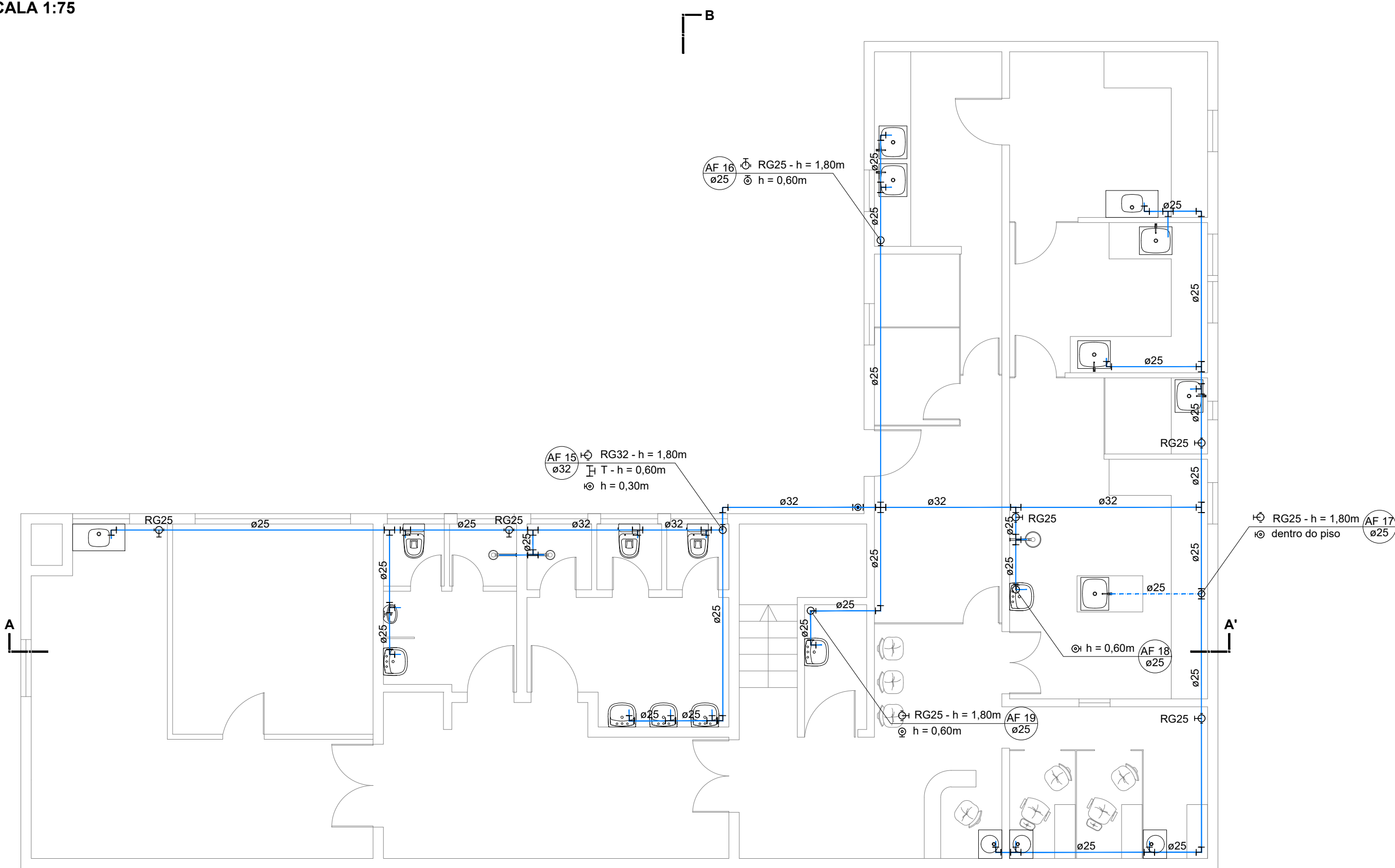
PLANTA BAIXA - TÉRREO ESCALA 1:75
