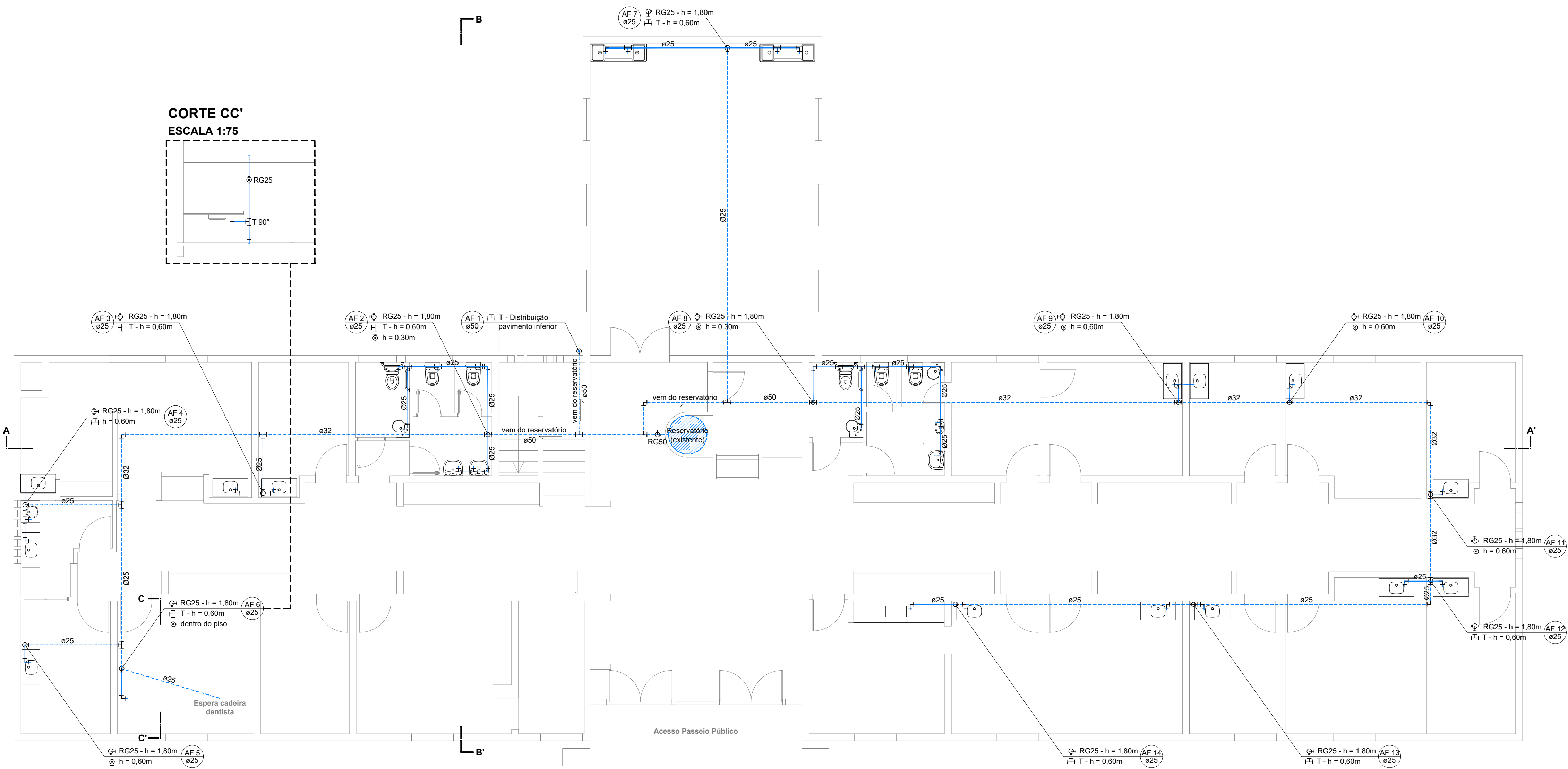
PLANTA BAIXA - TÉRREO ESCALA 1:75
