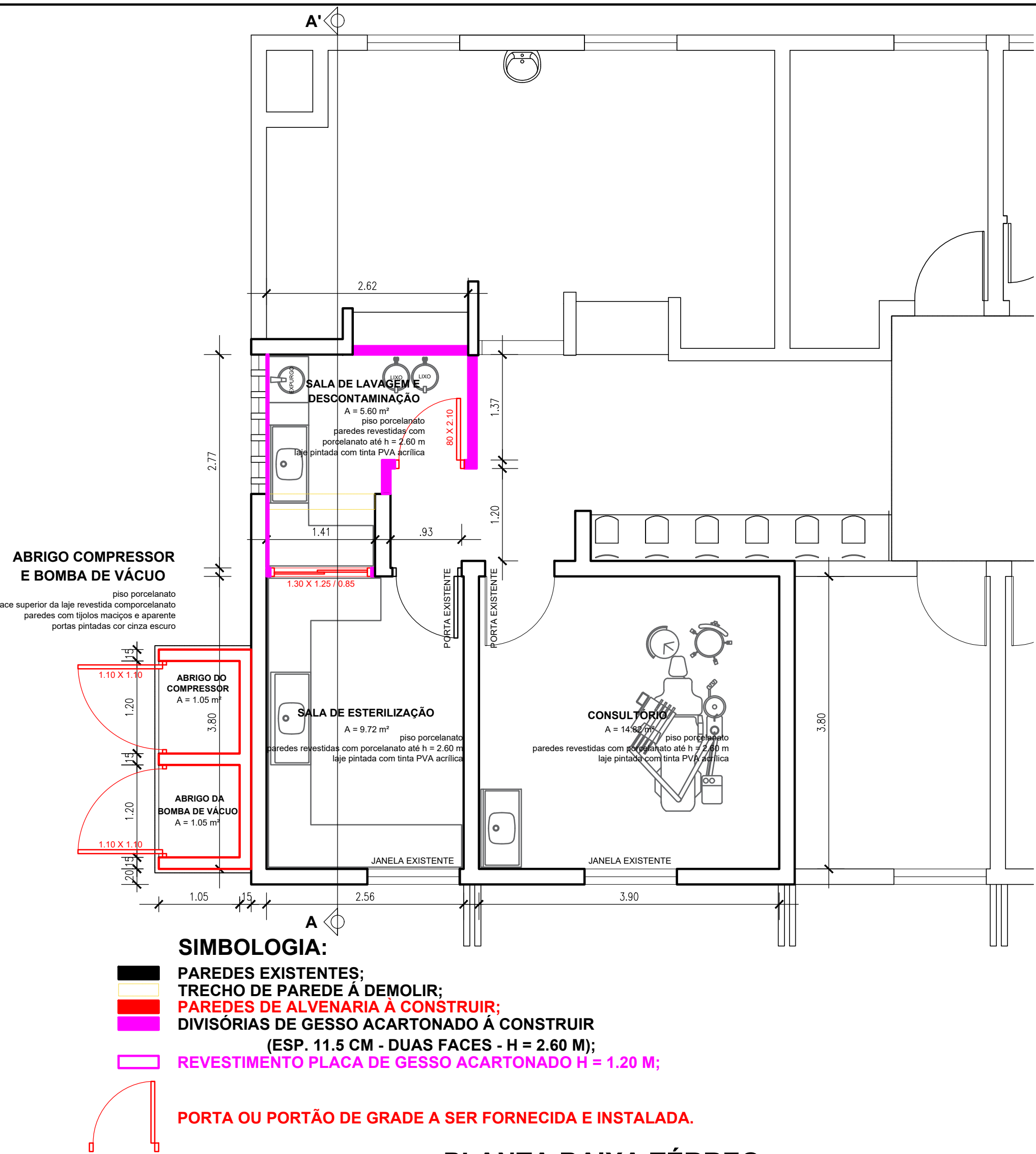
PLANTA BAIXA TÉRREO ÁREA - 32.24 m² ESCALA 1/50
