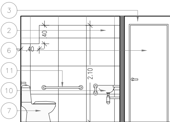
CORTE BB
