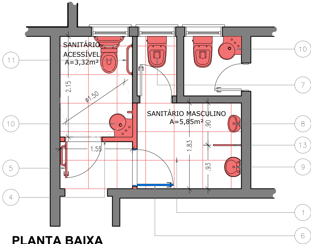
PLANTA BAIXA CONSTRUIR
